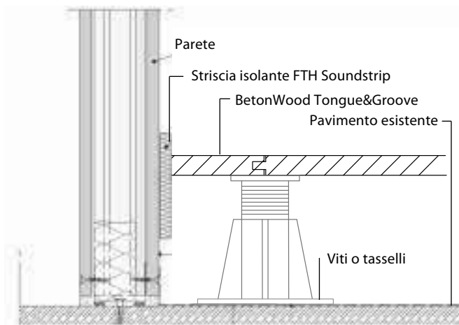
Collegamento con parete tramite strisce isolanti in fibra di legno FibberTherm Soundstrip
