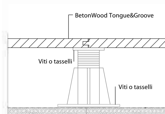
Corretto posizionamento dei supporti con livellamento a laser e fissaggio della testa con viti o tasselli
